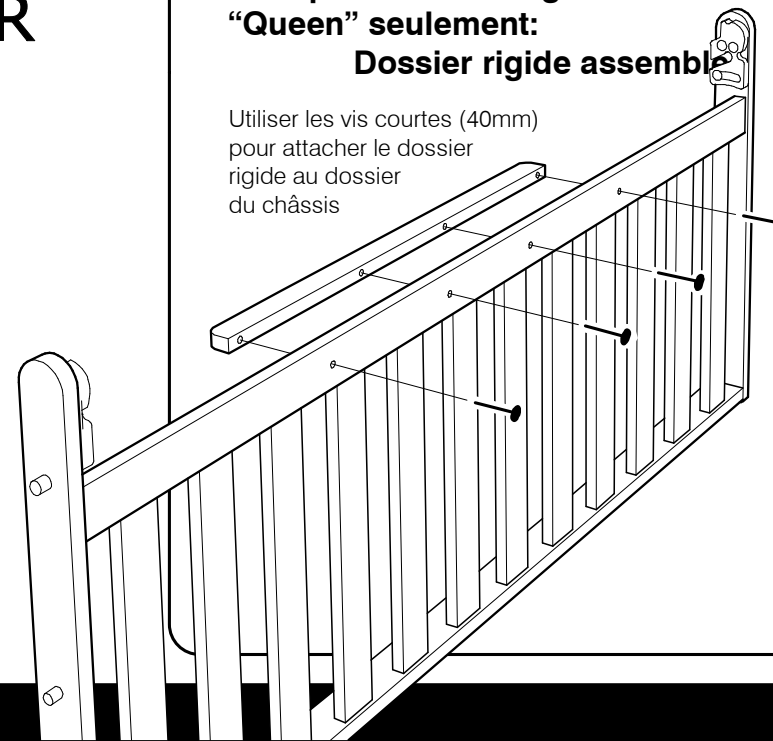
Vis (40mm) x 4
